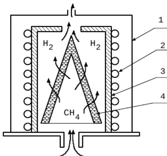
1 - кожух; 2 - индукционная катушка; 3 - графитовый сердечник; 4 - каркас из углеродистых нитей Рисунок 10 – Схемы осаждения углерода
